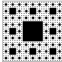
Alfombra de Menger d= 1,8928
