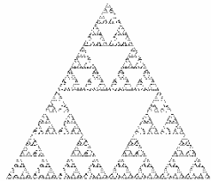
Triángulo de Sierpinski d=1,5850
