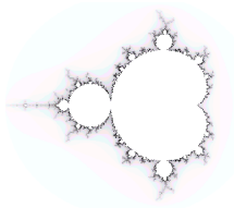
Conjunto de Mandelbrot d=2
