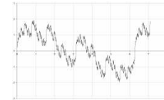
Función de Weierstrass d=1.5
