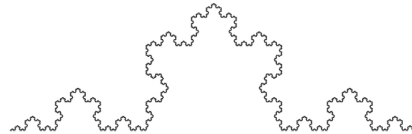
Curva de Koch d=1,2619
