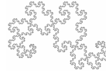
Curva de Dragón d=1,5236
