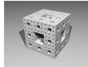
Esponja de Menger d=2,7268
