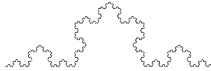
Curva de Koch d=1,2619
