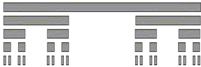
Conjunto de Cantor d=0,6309
