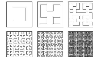
Curva de Peano d =2
