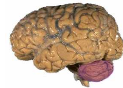
Superficie del cerebro d=2.79
